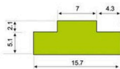
CADENA RODILLO 1/2
