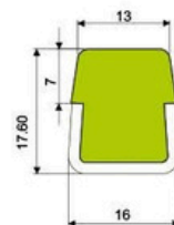
CÓNICO NEUMÁTICO
