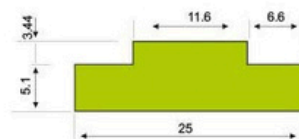
CADENA RODILLO 3/4
